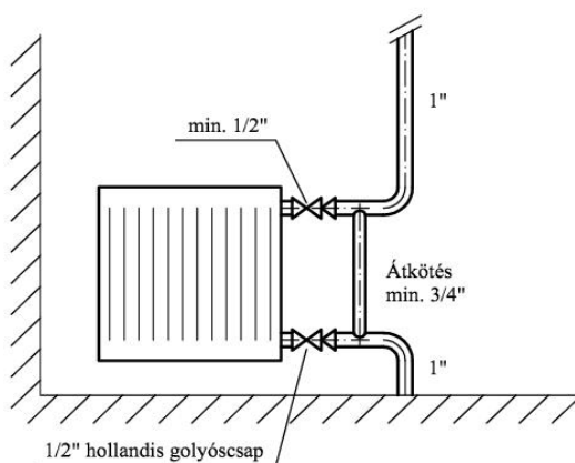
NAGYSZOBA
