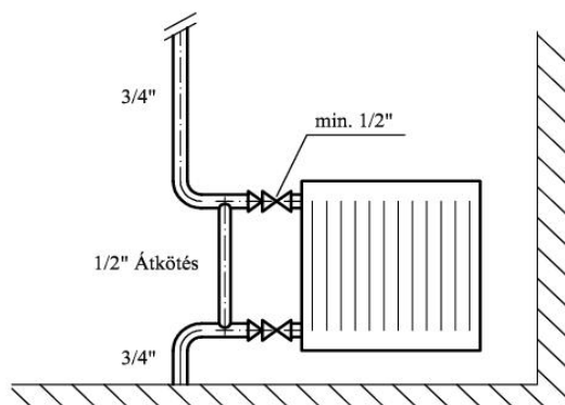
FÉLSZOBA 1
